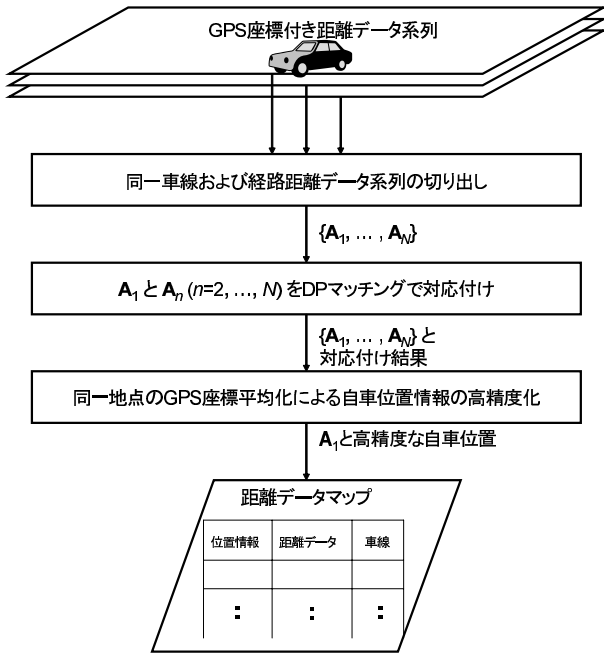
図5 距離データマップの構築手順
