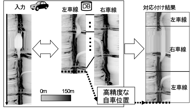
図6 入力距離データ系列と距離データマップとの対応付けの例
